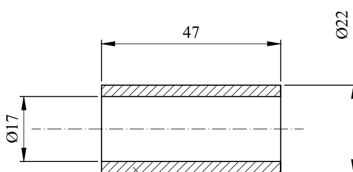
Teava Ø 22x2,5 EN 10219 - 2
