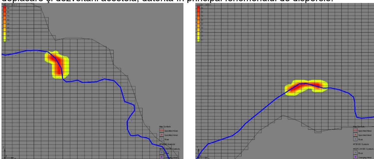
Figura 4.1.1.49 Situația privind dezvoltarea penei de poluant la 1 an de la începutul simulării
