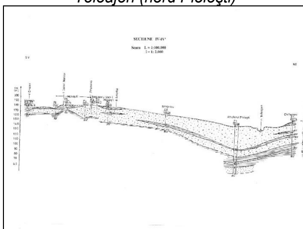
Figura 4.1.1.59 Secțiune hidrogeologică transversală prin conul Prahova Teleajen (sud Ploiești)
