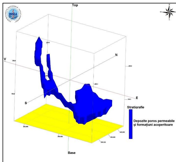
Figura 4.1.1.34 Model tridimensional al stratelor poros-permeabile din cadrul corpului de apă subterană ROIL12 – Câmpia Gherghiței
