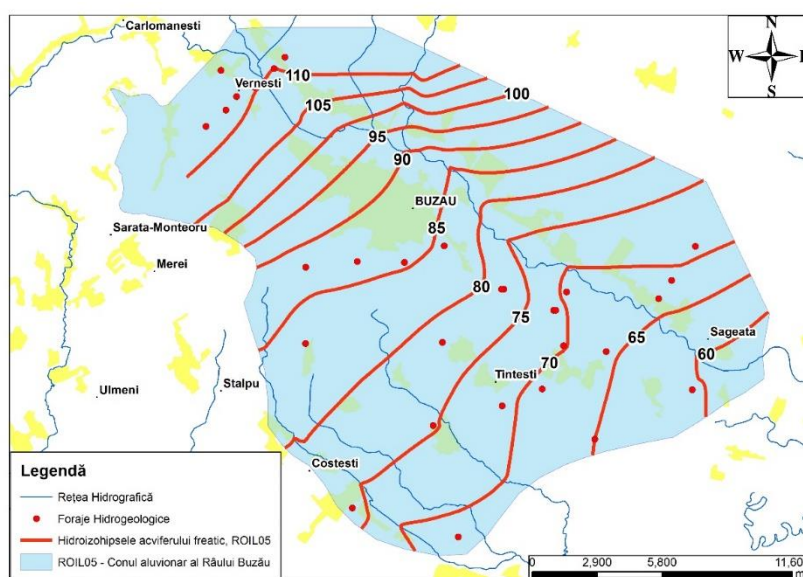
Figura 4.1.1.5 Spectrul hidrodynamic al acviferului freatic – corpul de apă subterană ROIL05
