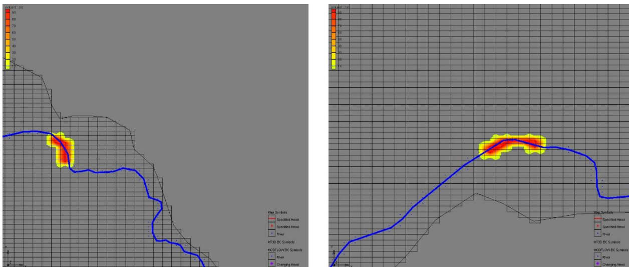
Figura 4.1.1.48 Situația privind dezvoltarea penei de poluant la începutul simulării
