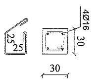
Sectiunea 1-1 scara 1:25
